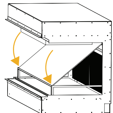
Afb. 9.3 | Zet glas in profiel aan voorzijde
