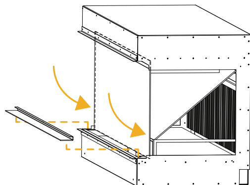
Afb. 9.5 | Zet glas recht en plaats opsluitprofiel
