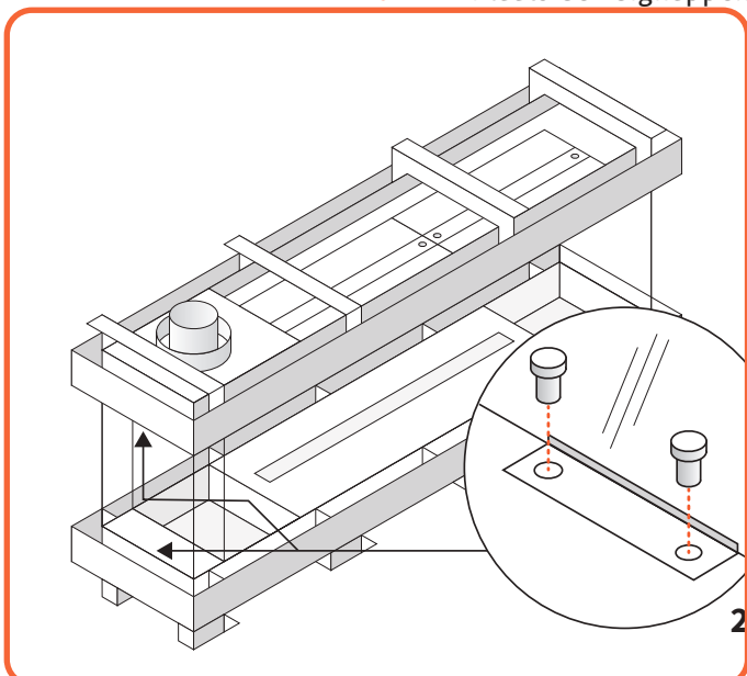
Afb. 9.19 Verwijder de glasklemmen aan de korte kant
