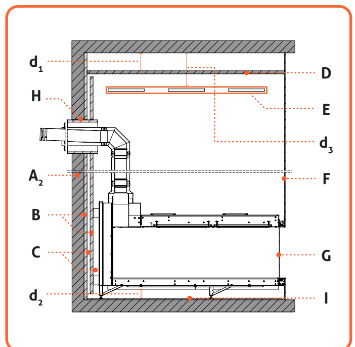
Afb. 6.4 C11: Gas afvoer bij brandbare materialen
