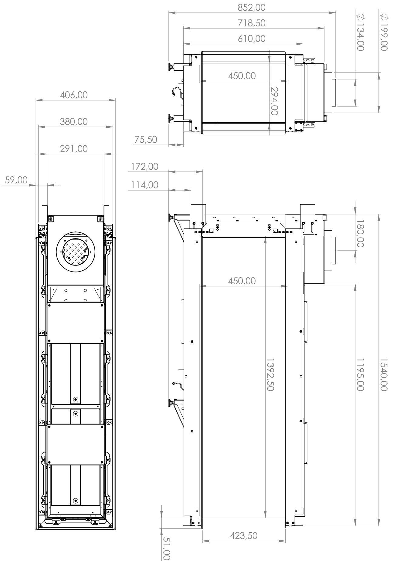
Afb. F.D Maattekening van de Summum 140 RD
