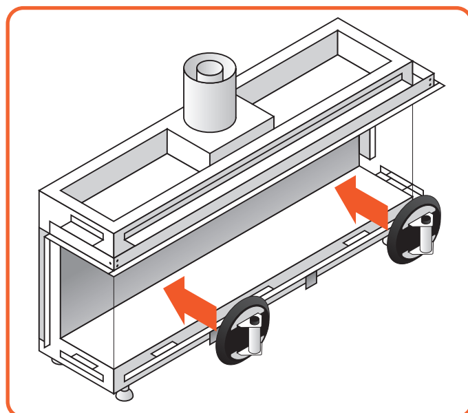
Afb. 9.5 Plaats de zuignappen
