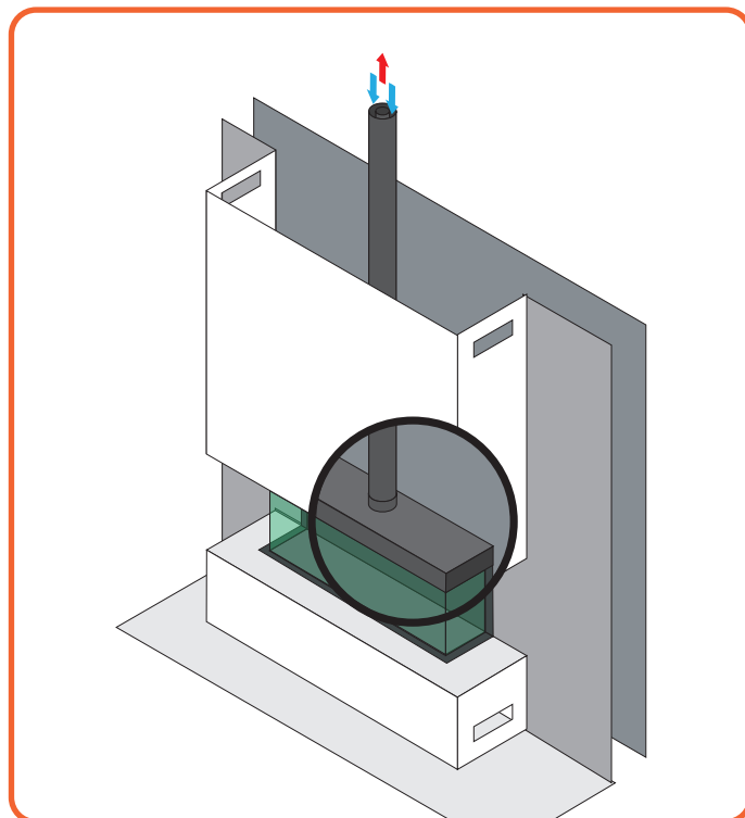
Afb. 5.3 Gebalanceerde aansluiting.
