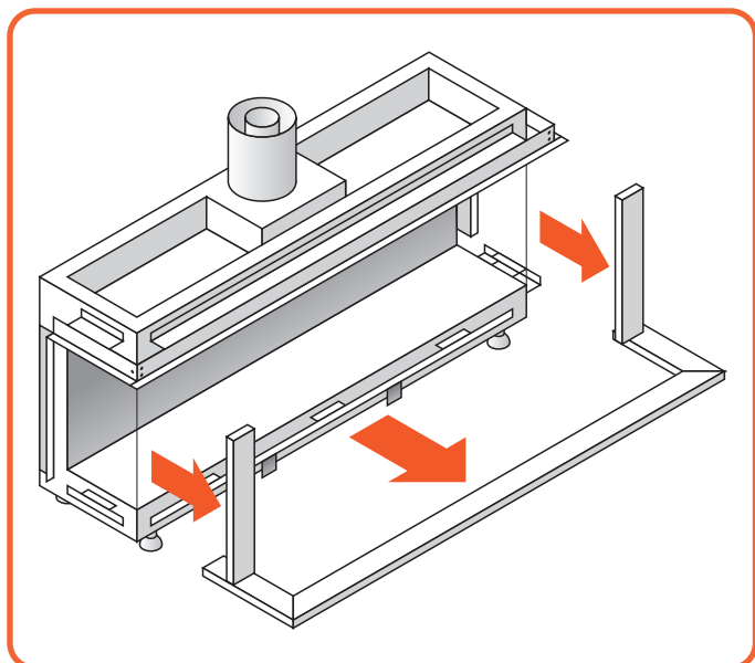
Afb. 9.3 Verwijder onderlijst
