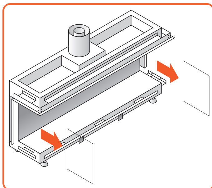
Afb. 9.7 Verwijder de zijglazen (indien nodig)
