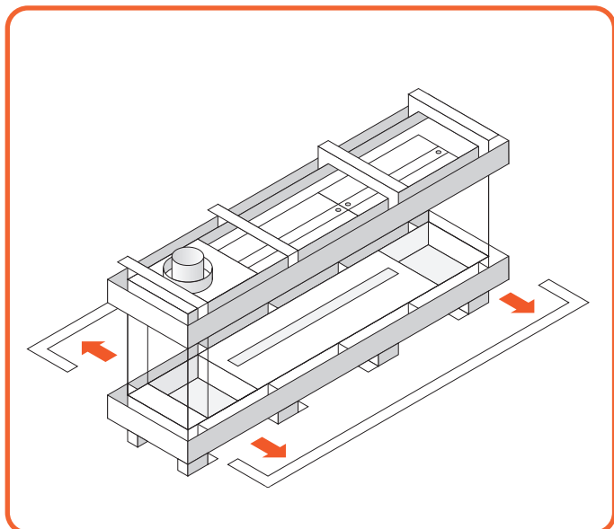
Afb. 9.15 Verwijder lijsten
