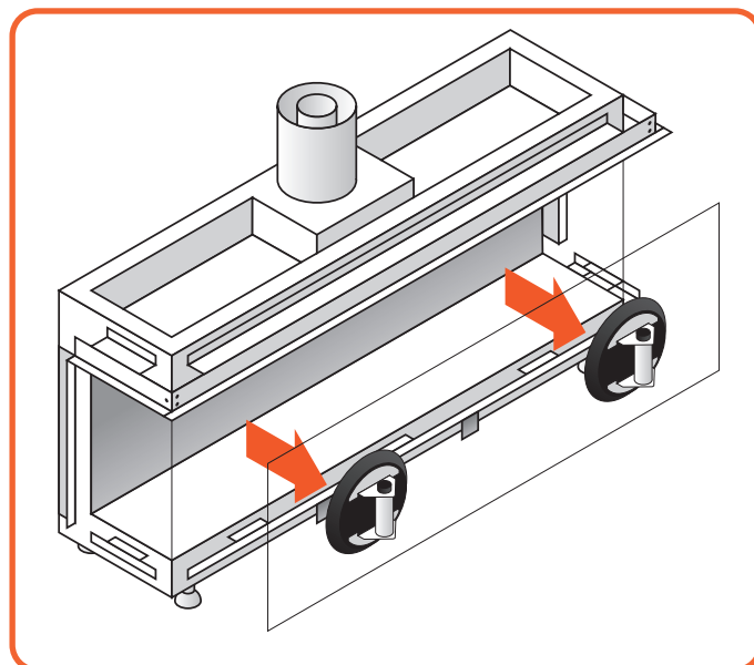
Afb. 9.6 Verwijder de glasplaat
