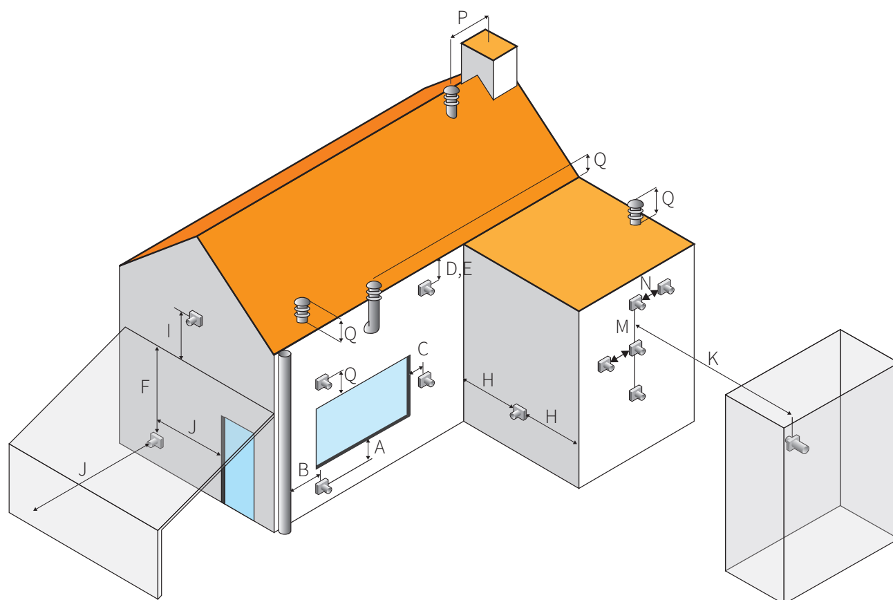
Afb. B.A Afvoerlocatie bij wandmontage
