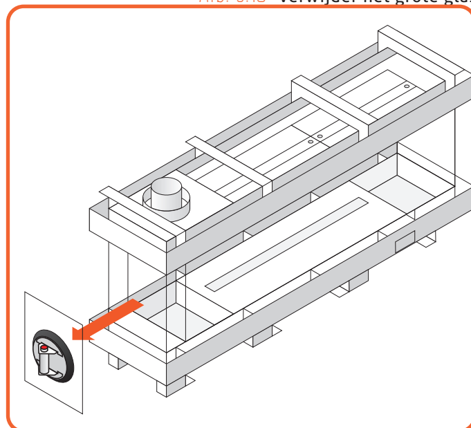
Afb. 9.20 Verwijder de zijruiten
