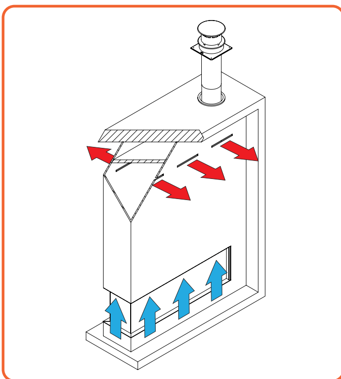
Afb. 6.6 Convectie uitlaat
