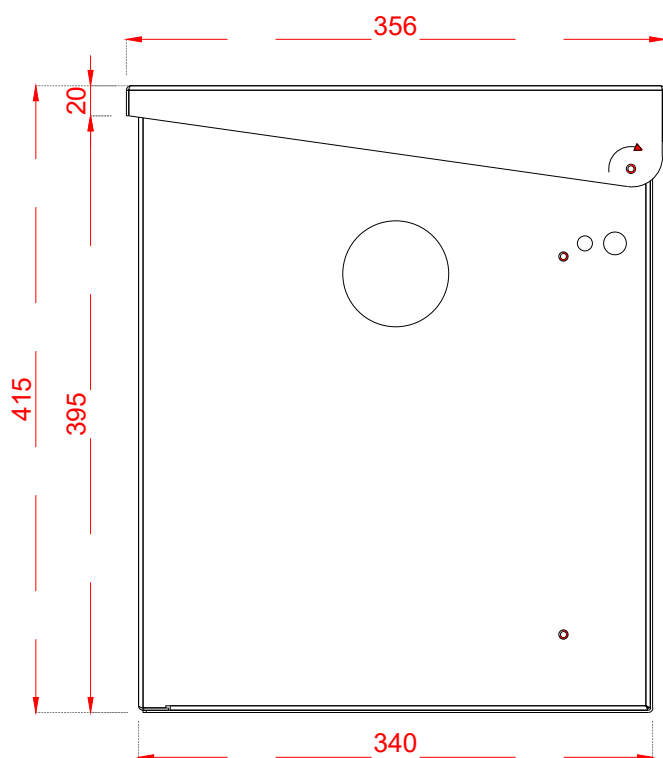
Rechterzijaanzicht
