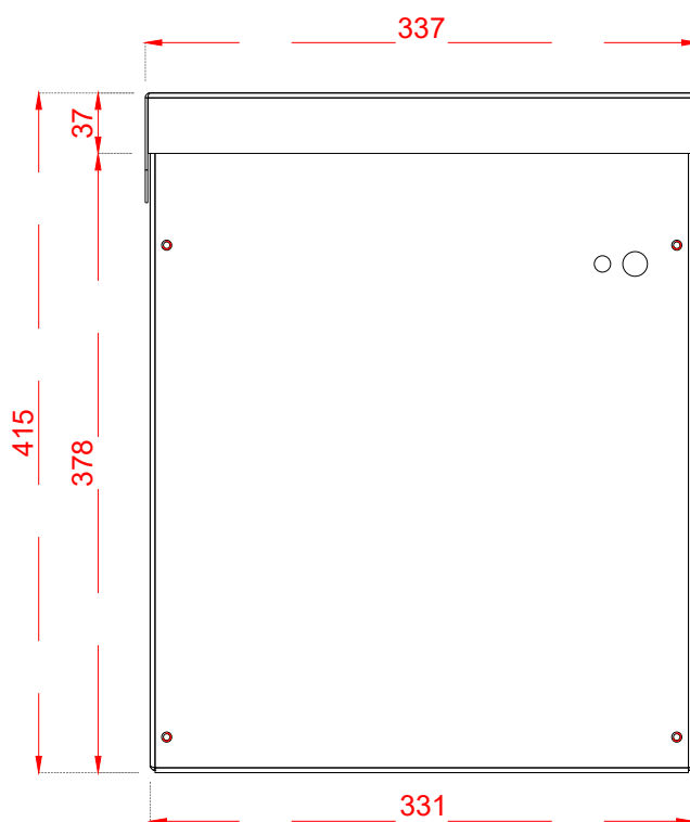
Achteraanzicht
