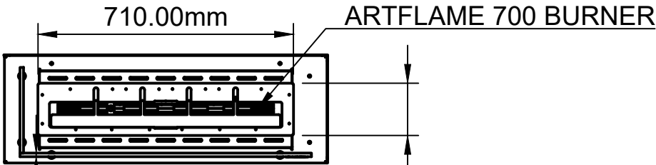
E-E (1:15)
