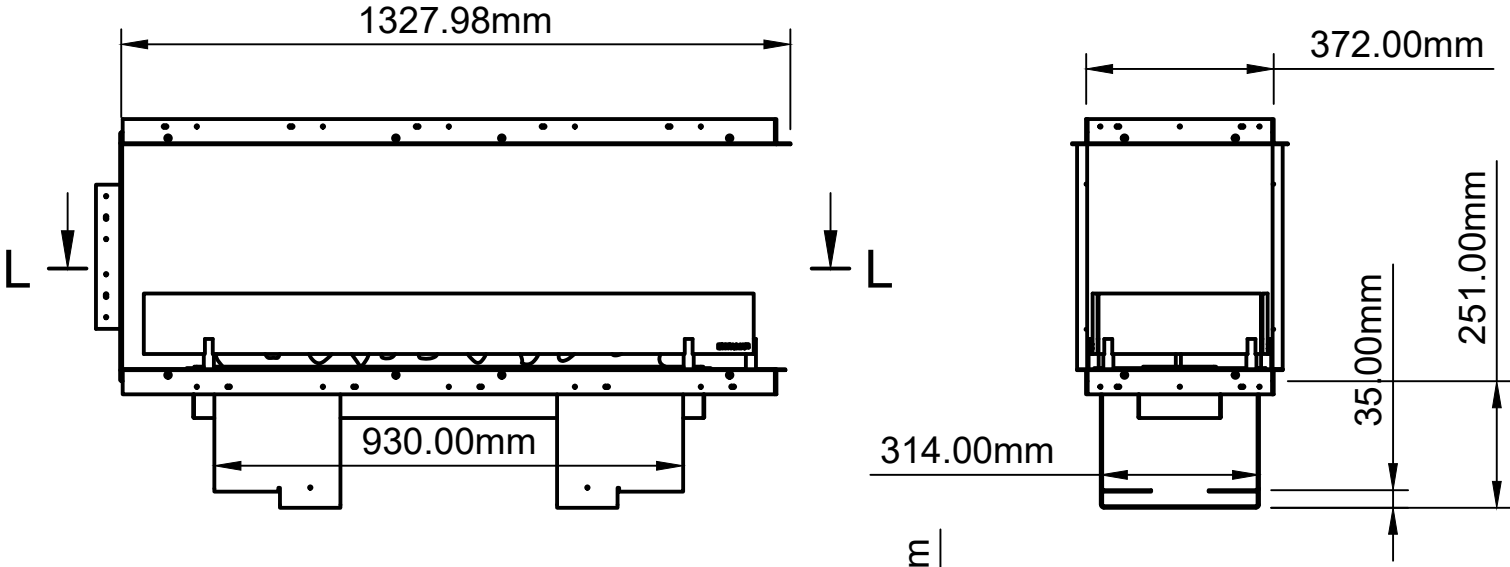
L-L (1:15)
